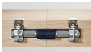
Conector para empalmes
